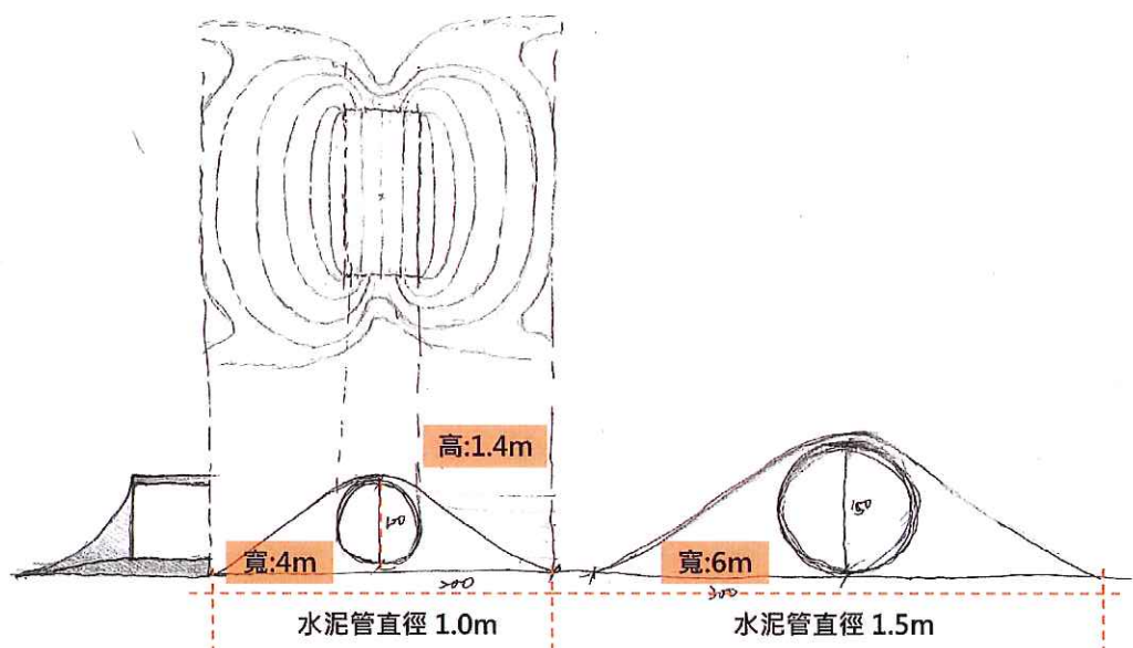
水泥管尺寸及等高線範例
